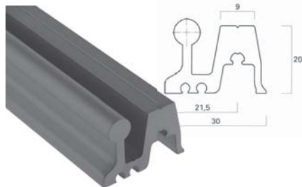
52.3410 Lodret vippeprofil
