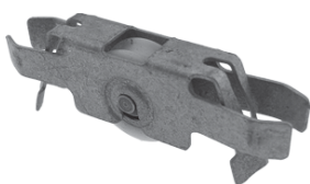
60.5050 Løberulle med stål kugleleje betrukket med nylonkappe. 2 stk. max 25 kg, 4 stk. max. 50 kg. glas.
